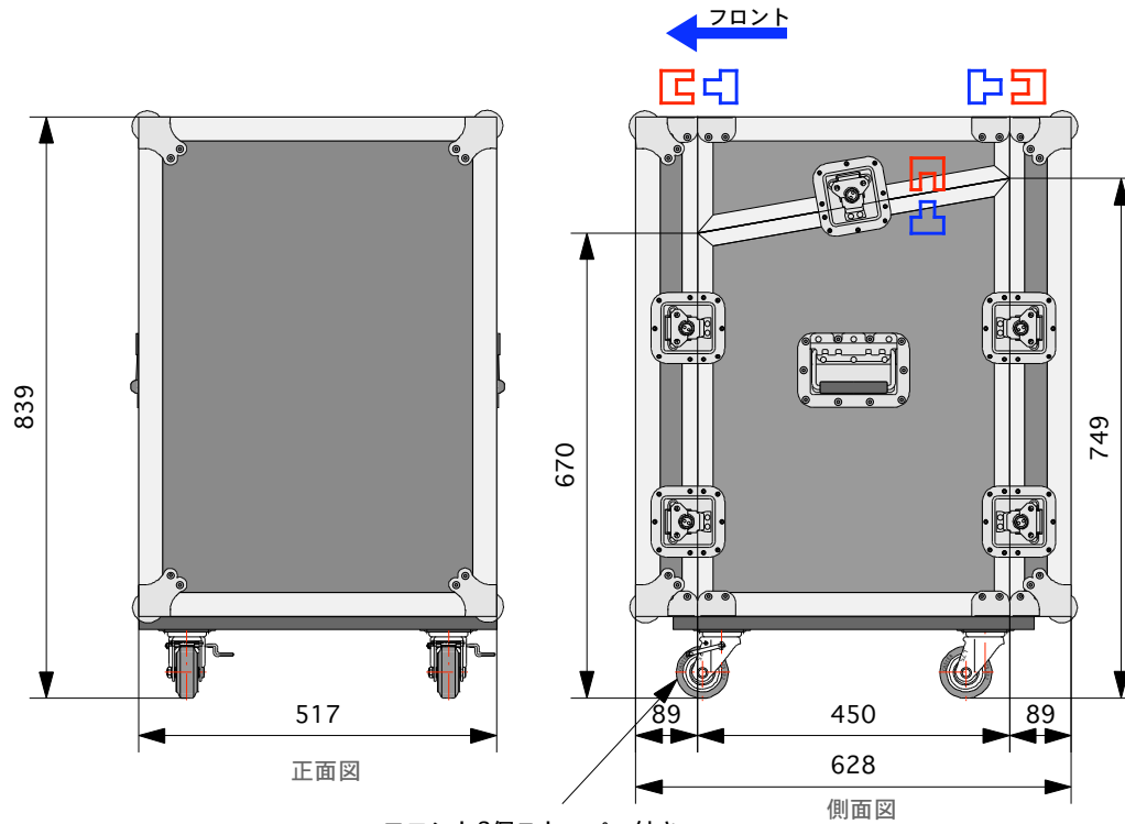
側面図
